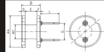
FIG(2) DRR-AxB-4C2H
