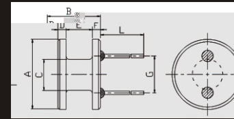
FIG(1) DRR-AxB-2H
